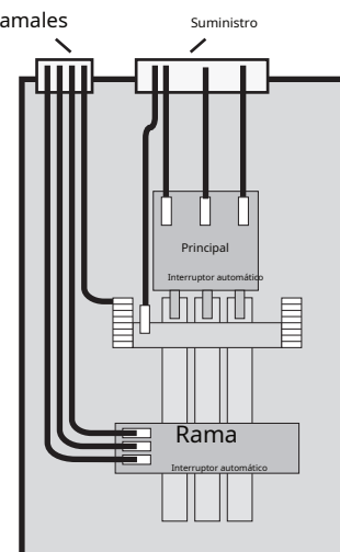
Interruptor principal montado verticalmente
