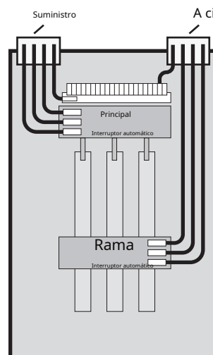
Interruptor principal montado horizontalmente
